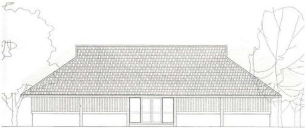
รูปด้านหน้าอาคาร ๑ : ๒๐๐
