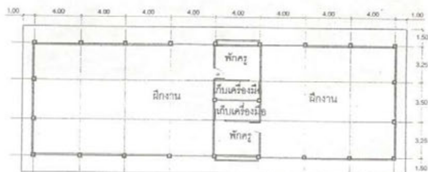
แปลนพื้น
